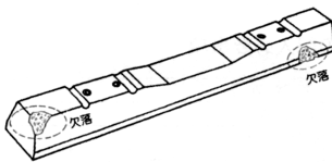
図 6.2.3 亀甲状および縦ひび割れ
