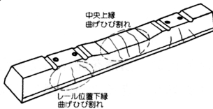
図 6.2.1 プレテンション方式の曲げひび割れ
