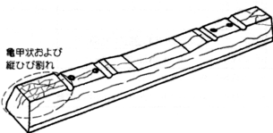
図 6.2.5 断面欠損
