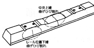
図 6.2.2 ポストテンション方式の曲げひび割れ
